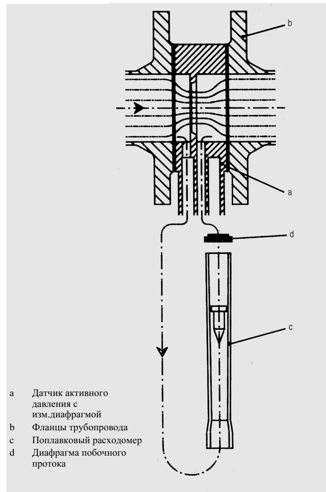
Рис 3/101 Принцип измерения
