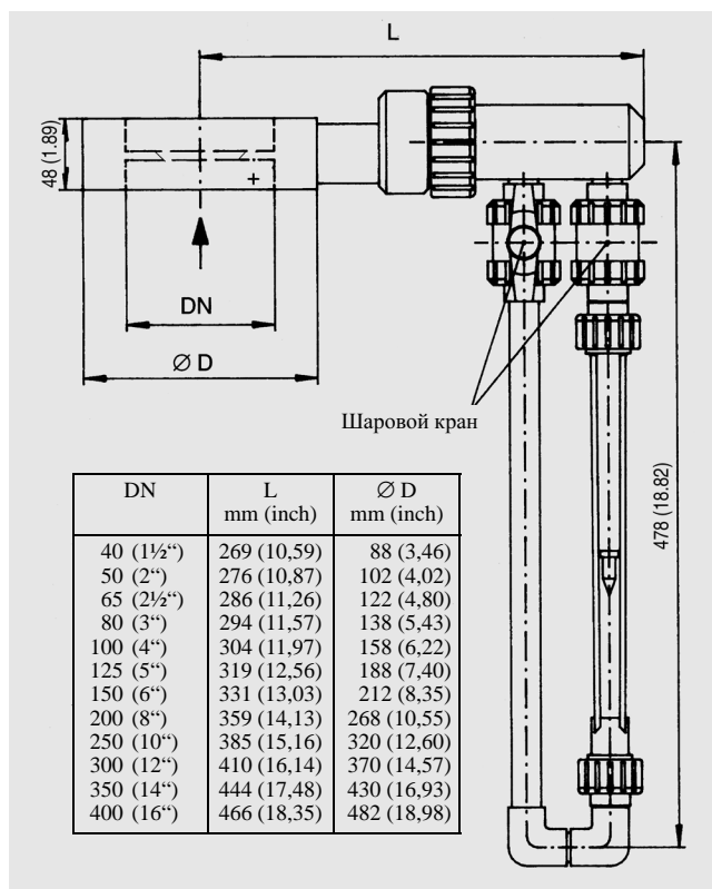
Рис 3/102 SITRANS FO N4, размеры в мм (inch)
